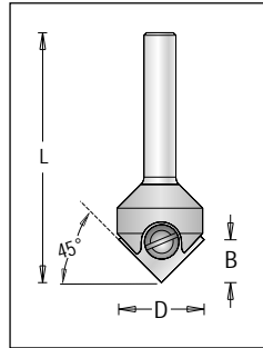
T.C Blade L12
